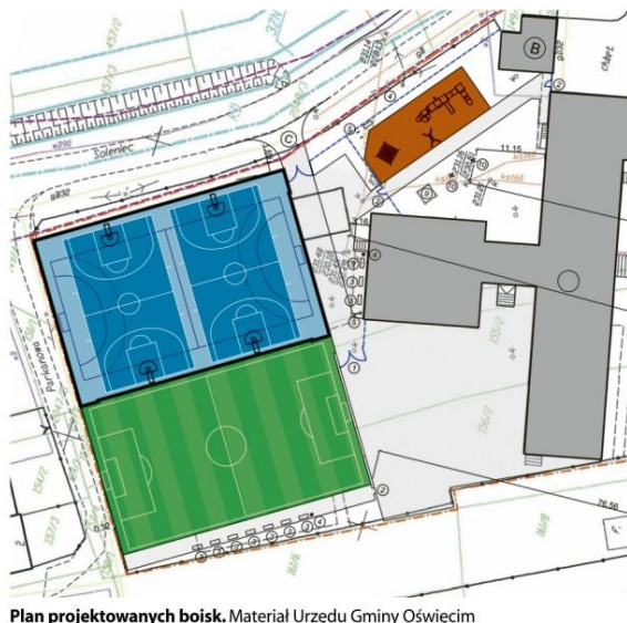
Plan projektowanych boisk. Materiał Urzędu Gminy Oświęcim
